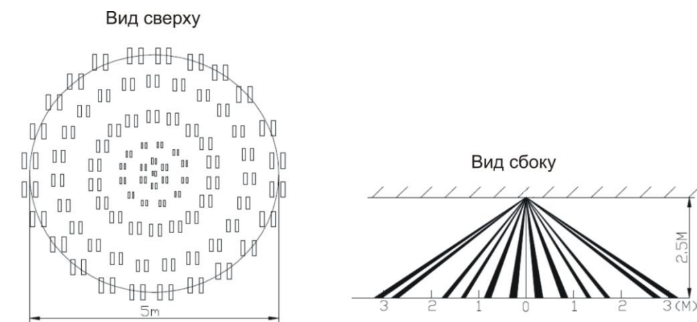
Рис. 2 Конфигурация зоны чувствительности датчика
