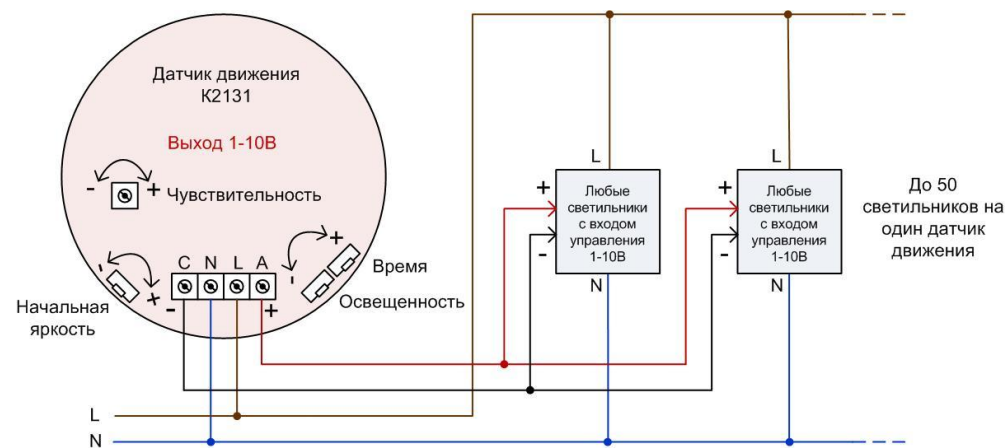
Рис. 1 Схема подключения датчика К2131
