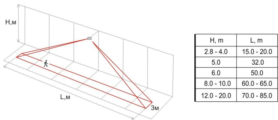
Рис. 4 Зона чувствительности датчика K2150 при установке на потолке внутри помещения
