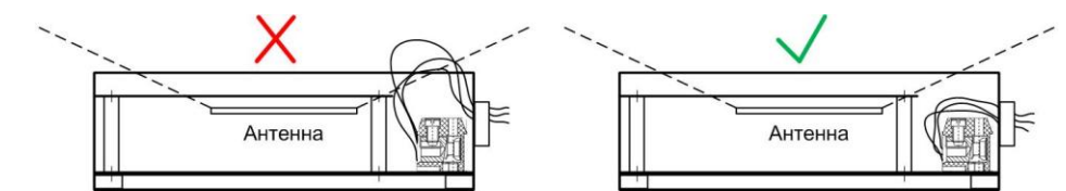
Рис. 3 Укладка проводов внутри датчика – уложите провода правильно!!!
