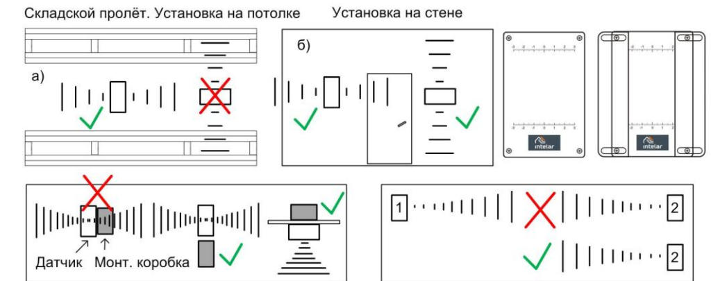
Рис. 2 Варианты установки датчика на потолке, стене и его внешний вид
