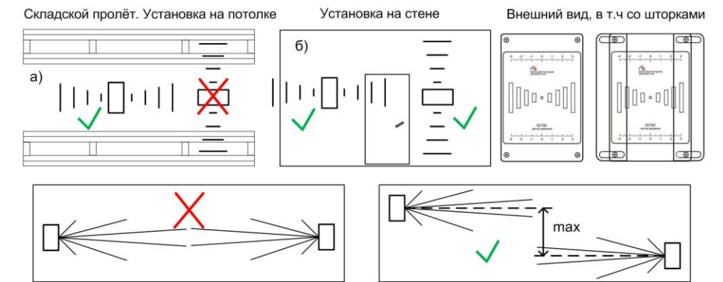
При креплении на стену не устанавливайте датчики друг напротив друга! Разнесите их максимально далеко. Рис. 2 Варианты установки датчика на потолке, стене и его внешний вид
